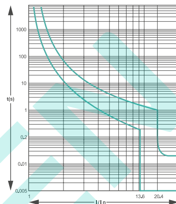
ХАРАКТЕРИСТИКА D
